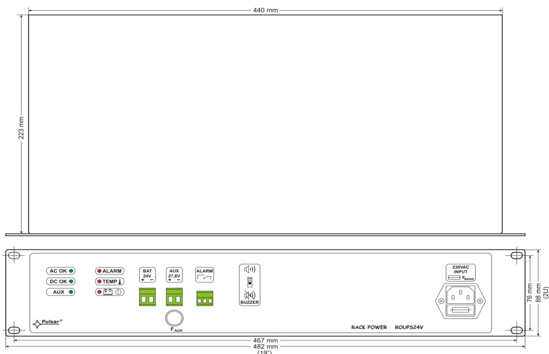
Rys.3. Widok zasilacza.
